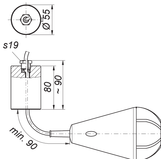
Lest FG 55x80/E en acier inox 316Ti
