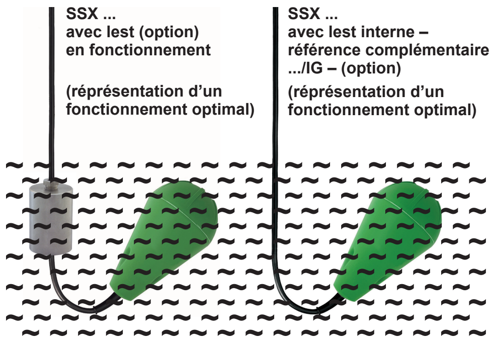
Lest FG 55x80/E en acier inox 316Ti
